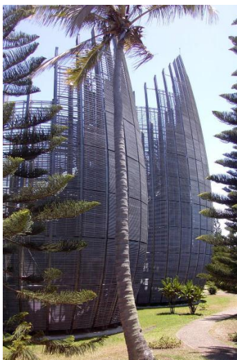
Ossatures lamellées-collées du centre culturel Jean-Marie Tjibaou - Nouméa, Nouvelle- Calédonie (photo J. Gérard).
